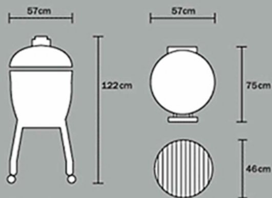
02 Корпус с подставкой
