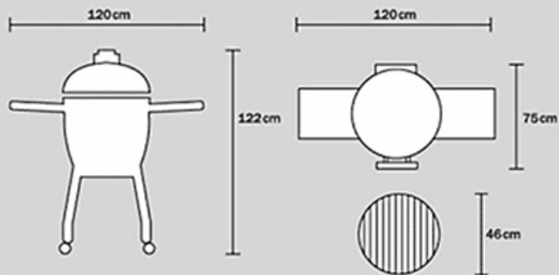
03 Корпус с подставкой и со столиком
