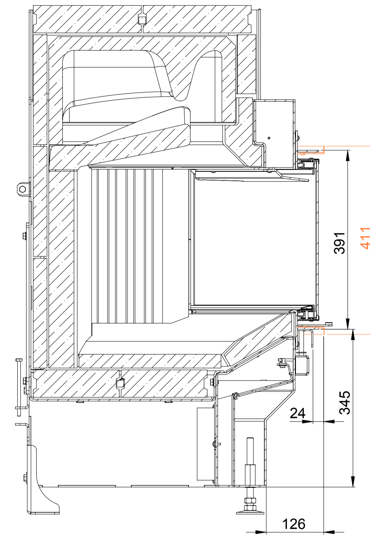
SCHNITT C-C
